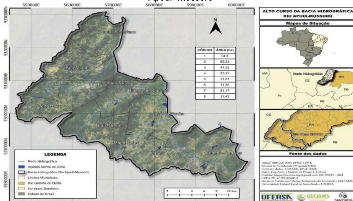
Figura 3 – Espelhos d'água superiores a 20 ha. no Alto curso da Bacia Hidrográfica do Rio Apodi- Mossoró
