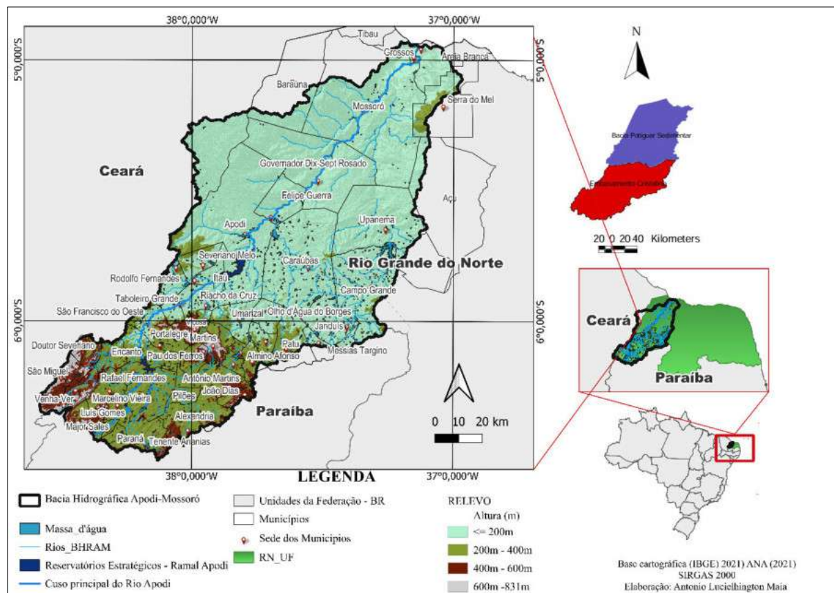
Figura 1 – Localização da Bacia Hidrográfica Apodi-Mossoró
