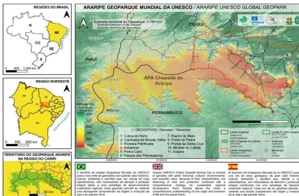
Figura 1 – Mapa do Geoparque Araripe e localização dos geossítios
